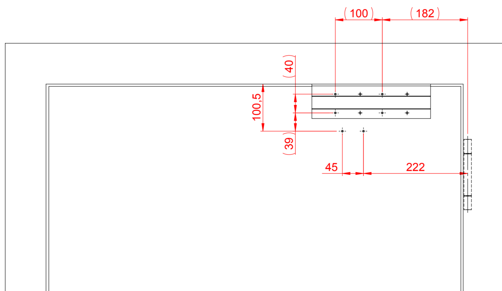
Anbauvariante Direktmontage EN 3 + Sturzfutterwinkel
