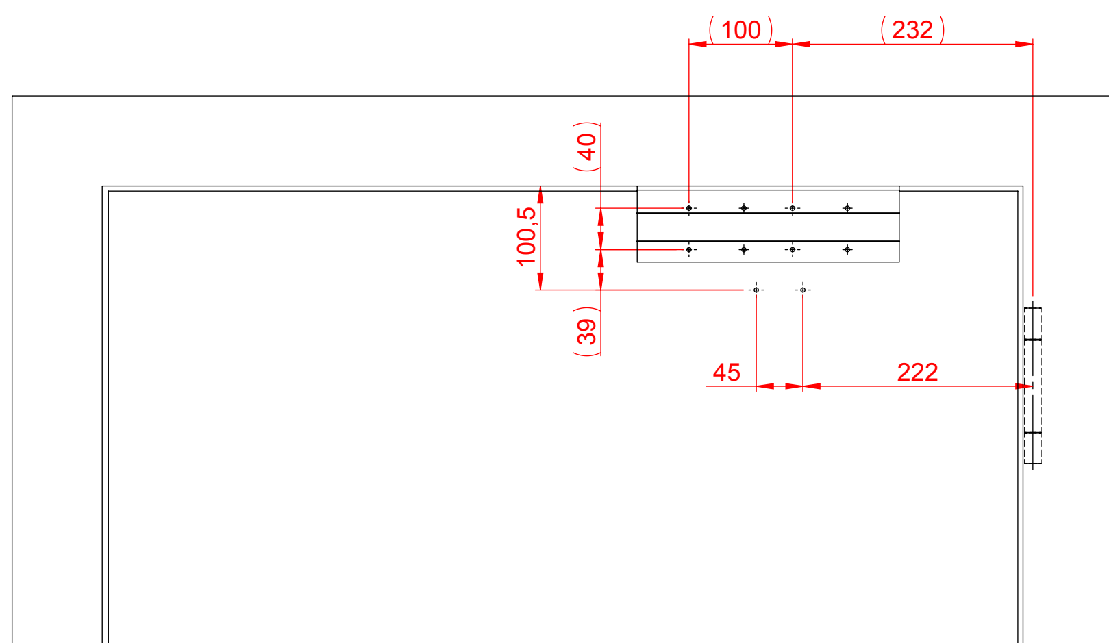
Anbauvariante Direktmontage EN 5 + Sturzfutterwinkel
