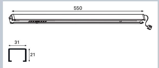
Montage glissière ECO IS EF
