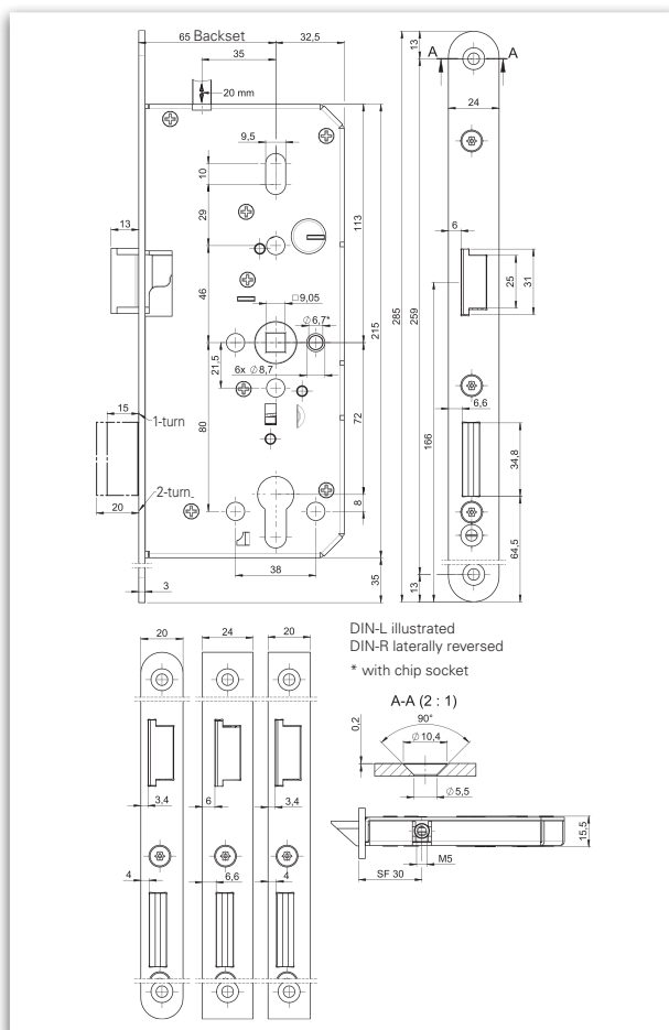
Dimensioning: GBS 130
