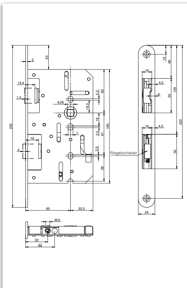
Bemaßung: GBS 94
