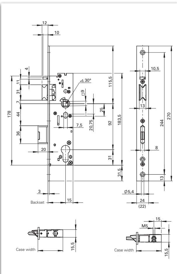
Dimensioning: GBS 96 AVP
